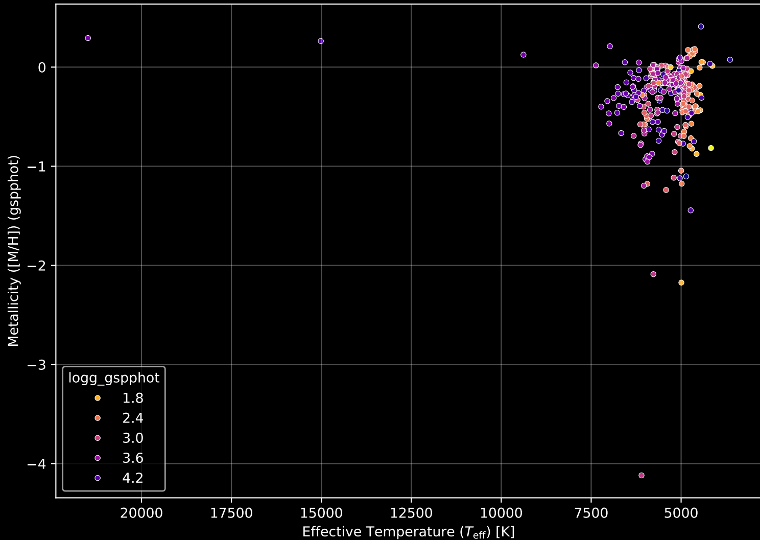
APOGEE DR17 Field: [M92] Stellar Population Parameters (n= 354)
